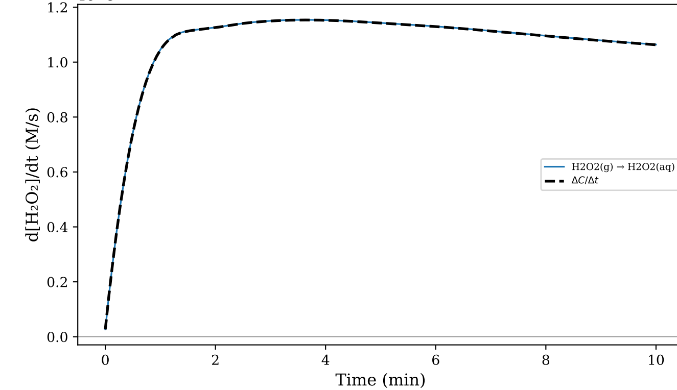
(d) \text{H}_2\text{O}_2
